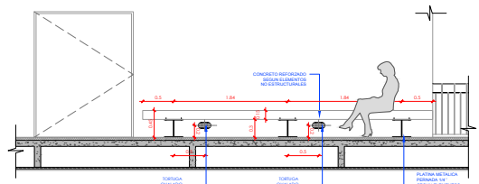
IMOBILIARIO BANCA TRIANGULO ESCALA 1:25
