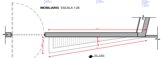
IMOBILIARIO BANCA TRIANGULO ESCALA 1:25
