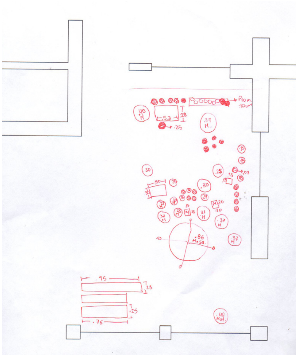
Materas de la oficina esquema en planta Office pots plan diagram
